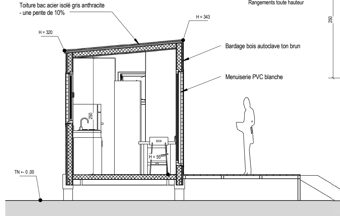
COUPE TRANSVERSALE
