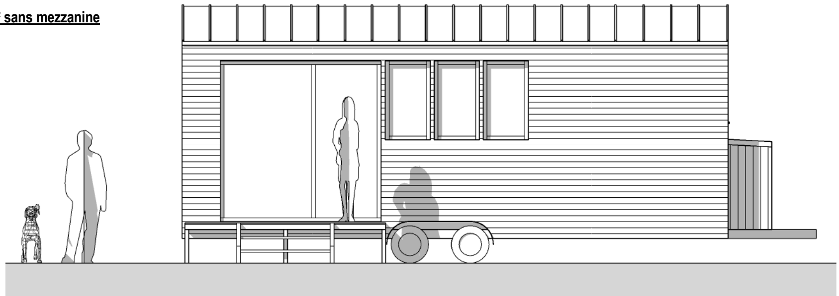
FACADE PRINCIPALE
