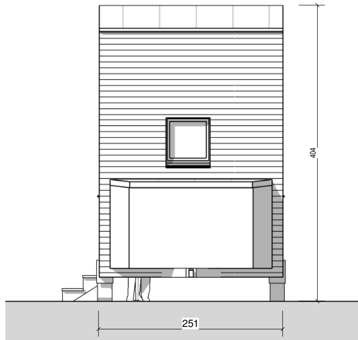
FACADE DROITE
