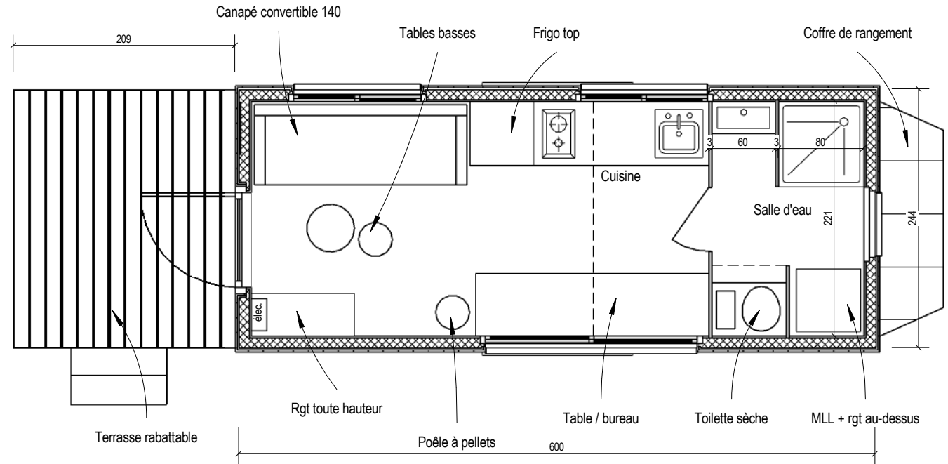
PLAN RDC
