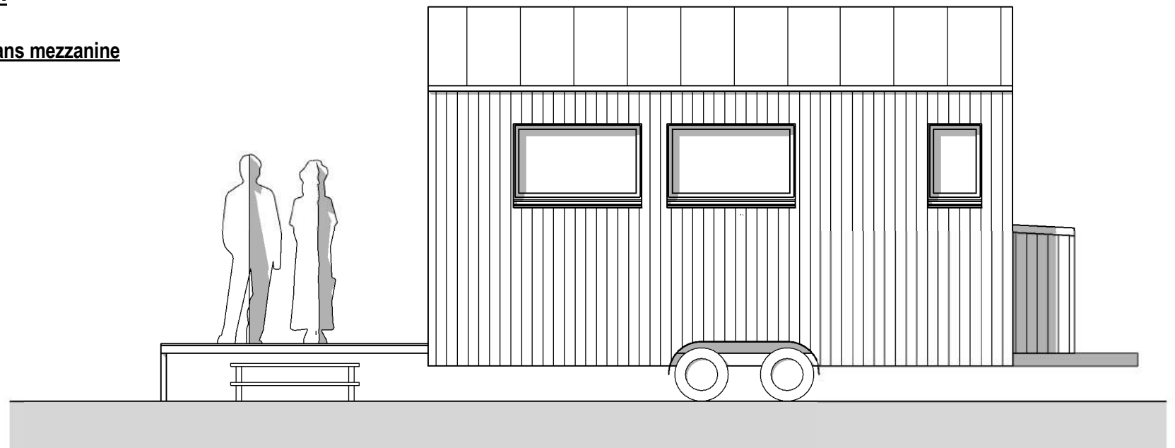
FACADE PRINCIPALE
