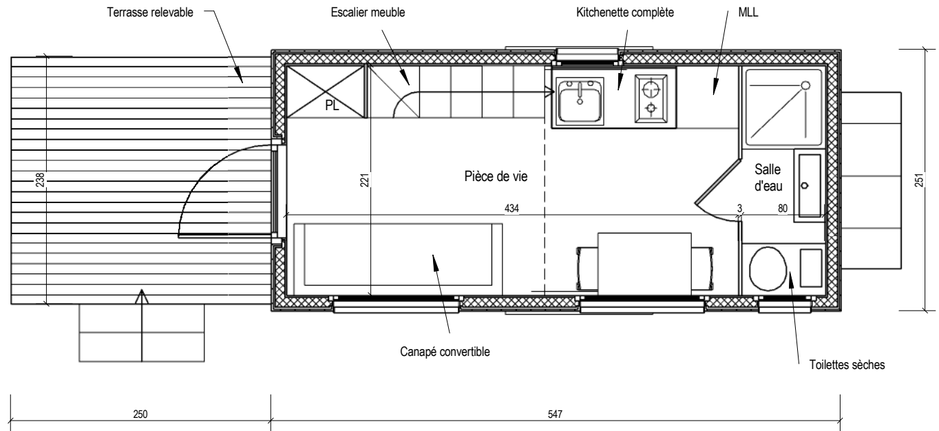
PLAN RDC
